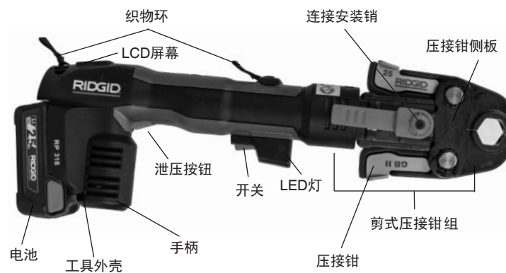
图1 - RP318压接工具和标准型压接钳组
